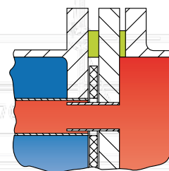
WRA 200, Détail du bouclier thermique
